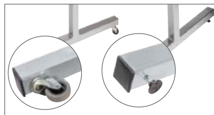
Piètement double en acier 40 x 40mm sur roulettes ou sur patins (intérieur)
